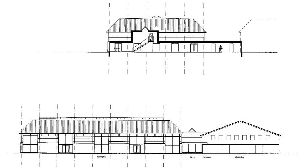
Snit i foyer og facade mod syd
